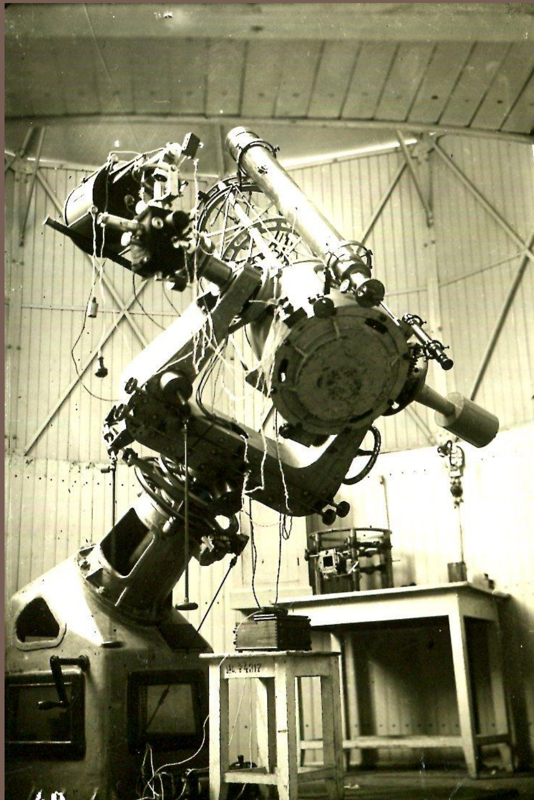
13-ти дюймовый рефлексор Пономарёва В Абастуманской обсерватории.
