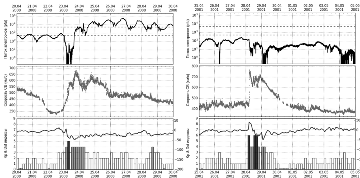
Рис. 2. Поведение потока высокоэнергичных электронов с энергиями более 2 МэВ на геостационарных орбитах во время межпланетных возмущений, вызванных высокоскоростным потоком из корональной дыры (левая панель) и корональным выбросом солнечной плазмы (правая панель).
