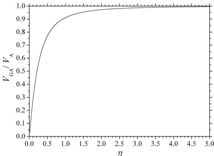
Рис. 1. Зависимость отношения групповой скорости альвеновских возмущений V_{GA} к альвеновской скорости V_A от \eta = 2\omega H/V_A .
