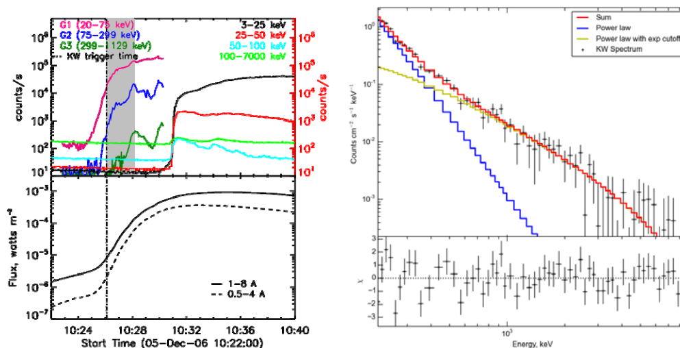
Рис. 3. Солнечная вспышка 2006/12/05 (X9.0). Слева: аналогично рис.2 и временные профили спутника RHESSI [6]. Справа: результат фитирования данных КВ двумя степенными функциями: степенная зависимость + степенная зависимость с экспоненциальным завалом в области высоких энергий.
