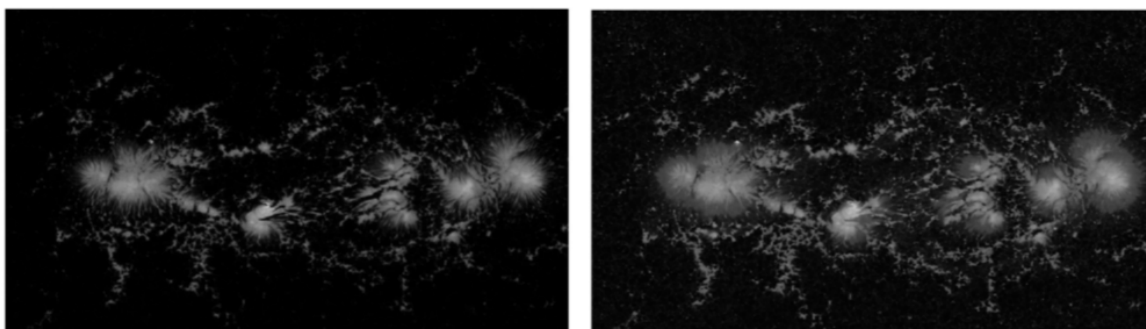
Рис. 4. То же, что и на рис. 3, для модуля вектора магнитного поля.
