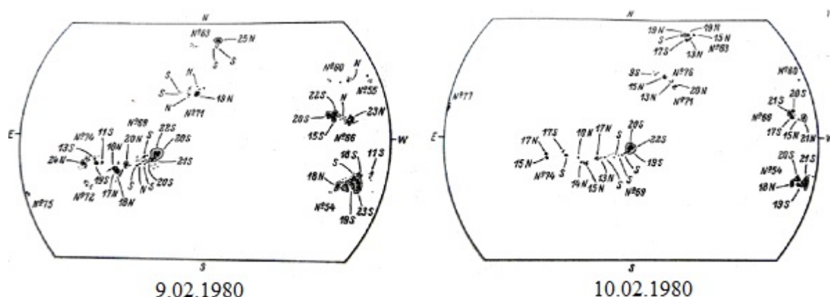
Рис.2. Карты магнитных полей солнечных пятен и изменения структуры групп пятен с 9 на 10 февраля 1980 по данным Кисловодской станции ГАС ГАО РАН (Солнечные данные. Бюллетень № 2, 1980 г.)
