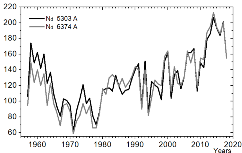
Рис. 3. Изменение количества дней корональных наблюдений за год.
