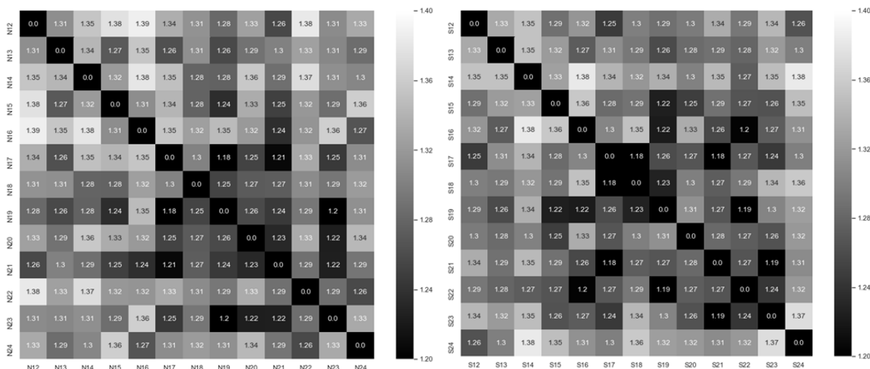
Рис. 3. Попарные расстояния между крыльями бабочек Северного (слева) и Южного (справа) полушариями Солнца, по осям отложены номера циклов (12÷24), более темный цвет означает более близкое расстояние.
