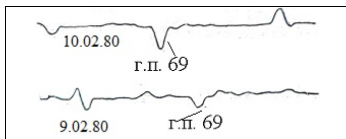
Рис.1. Упрощение записи поляризованного радиоизлучения Солнца на волне 2.3 см с 9.02. на 10.02.1980 г.
