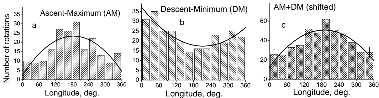
Рис. 2. Сильные поля ( B > 50 Гс): долготное распределение фотосферного магнитного поля в 1976–2016 гг. для интервала широт \pm 40^\circ ; а) фазы подъема и максимума СА; б) фазы спада и минимума; в) суммарное распределение для всех фаз солнечного цикла (суммирование гистограммы АМ со сдвинутой на 180^\circ гистограммой DM). Огибающие – аппроксимация полиномом второй степени.
