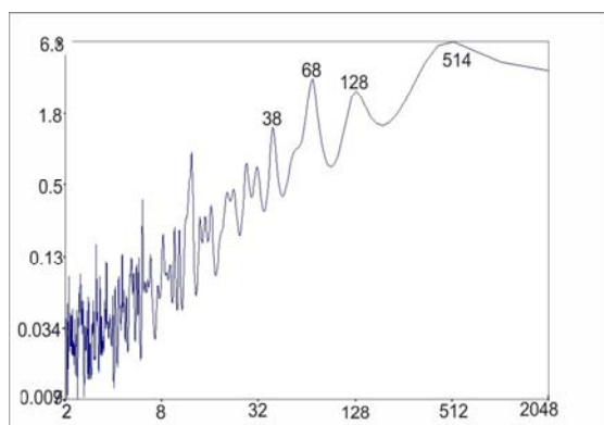
Рис. 3. Спектр мощности индекса PDO.
