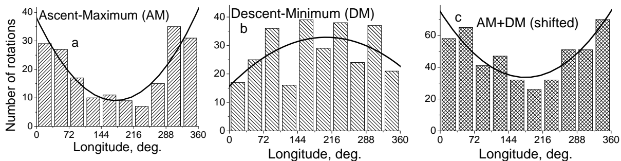
Рис. 3. То же, что на рис. 2 для слабых полей ( B < 5 Гс). Интервал широт \pm 90^\circ .
