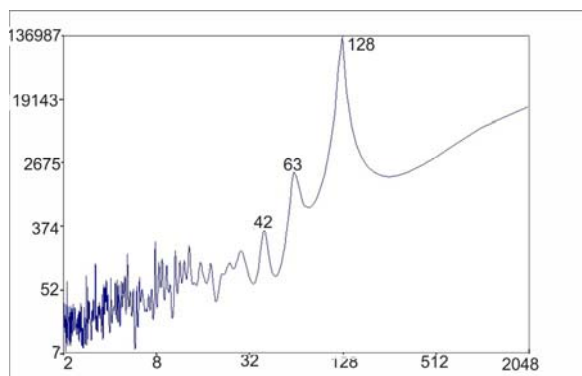
Рис. 1. Спектр мощности ряда числа солнечных пятен.
