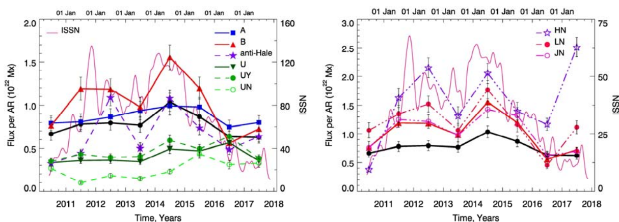
Рис. 3. Поток, приходящийся на АО данной группы, в зависимости от времени.
