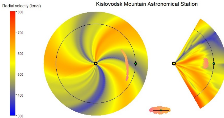
Рис. 1. Схема распространения солнечного ветра и КВМ.
