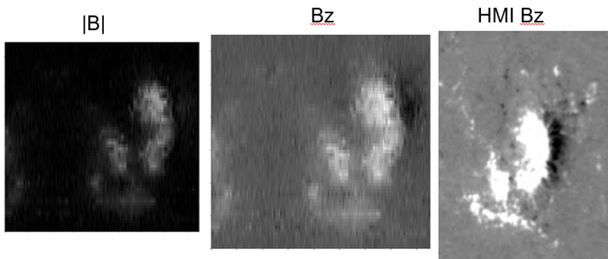
Рис. 5. Обработка данных, полученных на БСТ-1. Для сравнения справа приведена магнитограмма той же области, сделанная спутником HMI.
