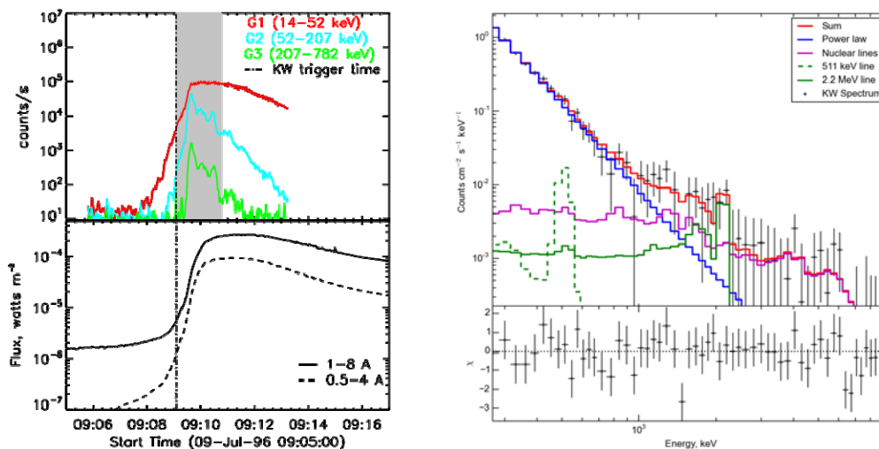
Рис. 2. Солнечная вспышка 1996/07/09 (X2.6). Слева: временной профиль жесткого РИ в трех каналах по данным КВ (верхняя панель), временной профиль мягкого РИ по данным GOES (нижняя панель). Справа: результат фитирования данных КВ четырехкомпонентной моделью, включающей степенную функцию, шаблон излучения в ядерных линиях, линию аннигиляции электрона и позитрона 511 кэВ и линию захвата нейтрона 2.2 МэВ.
