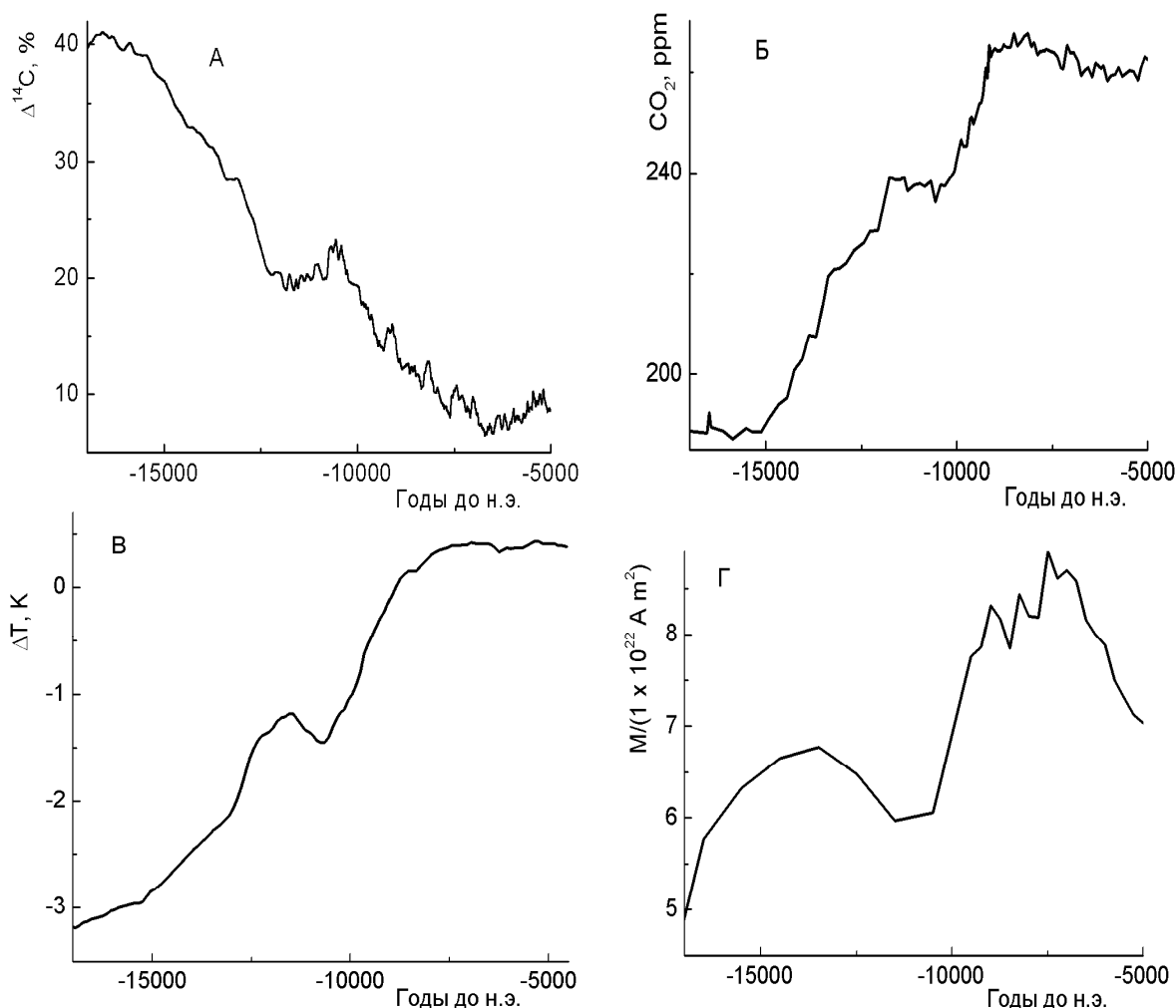
Рис. 1. А – Вариации \Delta^{14}\text{C} в атмосфере Земли [1]; Б – Изменение концентрации углекислого газа в земной атмосфере [2]; В – Изменение глобальной приземной температуры [3, 4]; Г – дипольный магнитный момент Земли [7].
