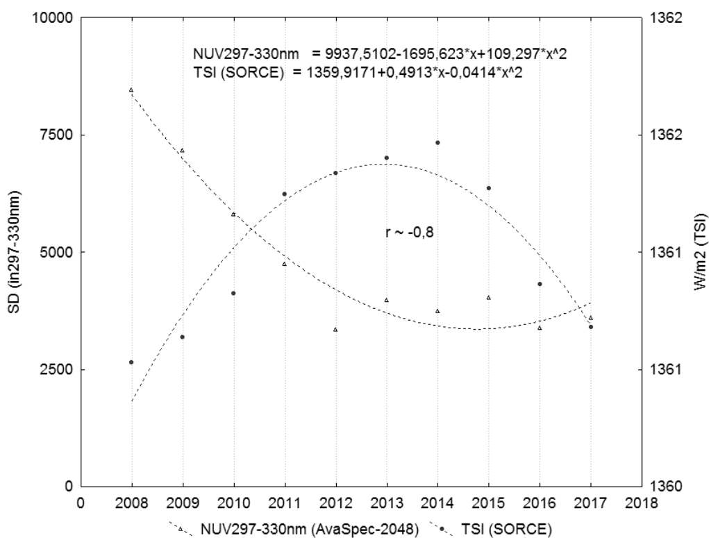
Рис. 1. Сравнение среднесезонных (сентябрь–февраль) значений излучения NUV 297–330 nm по данным AvaSpec-2048 (ст. Новолазаревская) и общей солнечной радиации (TSI) по данным http://lasp.colorado.edu/sorce в 24-м цикле солнечной активности
