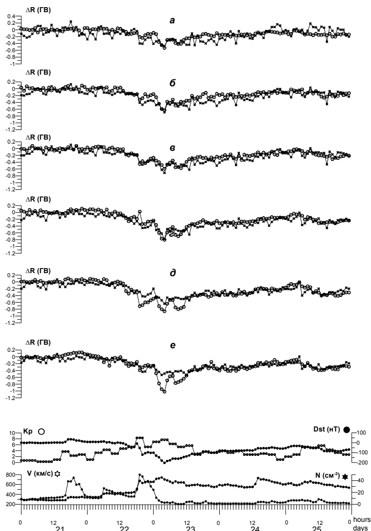
Рис. 1. Жесткости обрезания космических лучей в период бури 21–25.06.2015 ( \Delta R_{\text{эф}} 01 – кружки, \Delta R_{\text{СГС}} – крестики), а – ESOI, б – Алматы, в – Рим, г – Иркутск, д – Москва, е – Кингстон.
