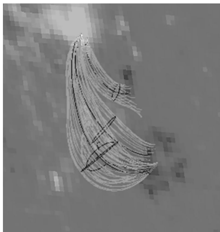
Рис. 1. Фоновое изображение – магнитограмма HMI/SDO и магнитные петли, полученные методом LFFF. Север – в верхней части рисунка.
