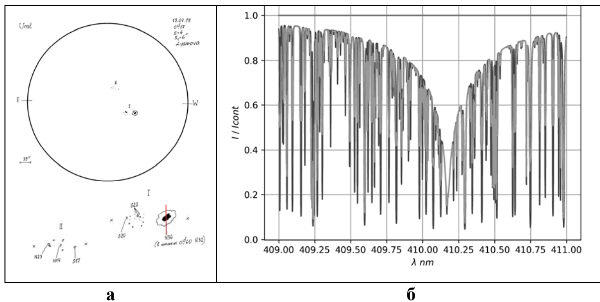
Рис. 1. а – сводка наблюдений МП солнечных пятен. Обозначено положение щели спектрографа; б – синтезированный по изложенной в статье методике спектр пятна в области линии H\delta , модель большого пятна согласно [10]. Черное – без МП, серое с МП 3600 Гс. Линии с МП шире и менее глубоки.
