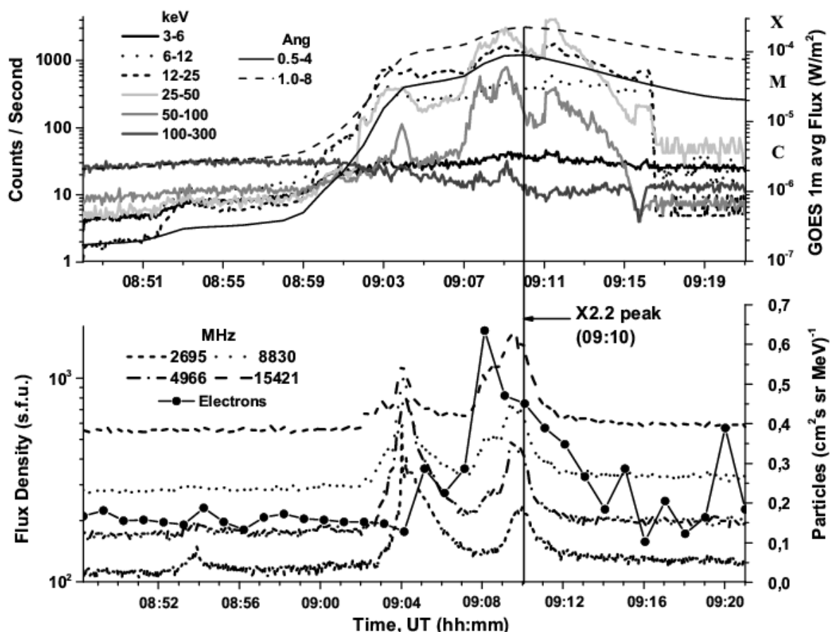
Рис. 1. Временные профили вспышечного излучения и зарегистрированные ускоренные электроны в событии X2.2 6 сентября 2017. Вверху: поток усред. за 1 мин. SXR-излучения (GOES, штриховая и сплошная плавные линии), HXR-всплеск (RHESSI, сплошная, пунктирная, штриховая кривые в каналах с энергиями 3–6, 6–12 и 12–25 кэВ; линии в градации серого – излучение в каналах 25–50, 50–100 и 100–300 кэВ). Верт. шкалы – значения потока W/m^2 , буквы – соответствующий балл (справа) и скорость счета в секунду (слева). Внизу: запись всплеска на микроволнах (RSTN, штриховая, пунктирная, штрихпунктирная и коротко-штриховая линии запись на частотах 15.4, 8.83, 4.96 и 2.69 ГГц), количество ускоренных электронов на единичную площадку в секунду с МэВ-энергией (SOHO/EPHIN, черные точки на кривой). Верт. шкалы – плотность потока в s.f.u. (слева, 1 \text{ s.f.u.} = 10^{-22} \text{ W m}^{-2} \text{ Hz}^{-1} ) и количество частиц (справа). Шкалы внизу: время в UT часах и минутах (чч:мм), соответственно. Верт. прямая линия – время пика вспышки по данным GOES.
