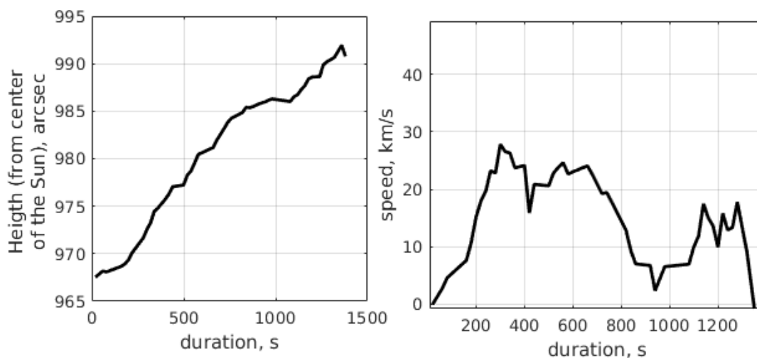
Рис. 3. Слева: смещение положения SXR (7–12 кэВ) источника во времени. Справа: скорость смещения источника во времени.
