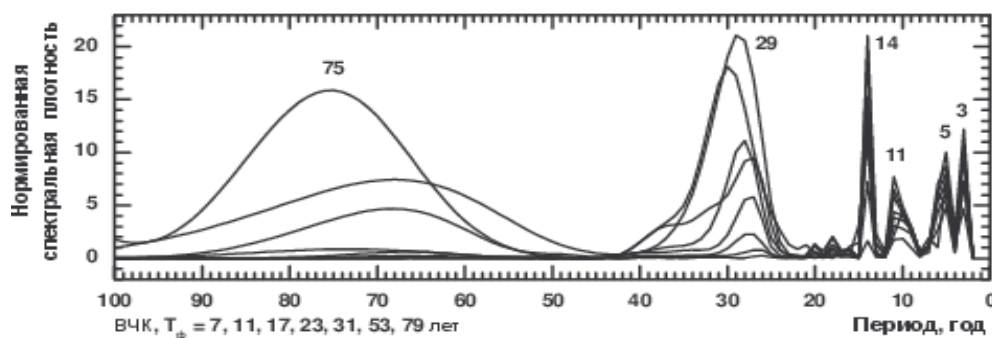
Рис. 2. КСП исходных палеоданных и их высокочастотных компонентов.
