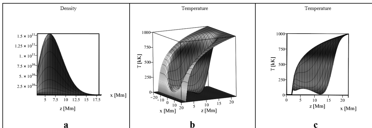
Рис. 2. а) Высотный профиль распределения плотности, б) трехмерный профиль температуры, с) высотный профиль температуры магнитной конфигурации (10), при следующих выбранных параметрах: B_0 = 6 Гс, k = 1/8 \text{Mm}^{-1} , z_0 = 2 Мм, \alpha = 0.27 \text{Mm}^{-1} .
