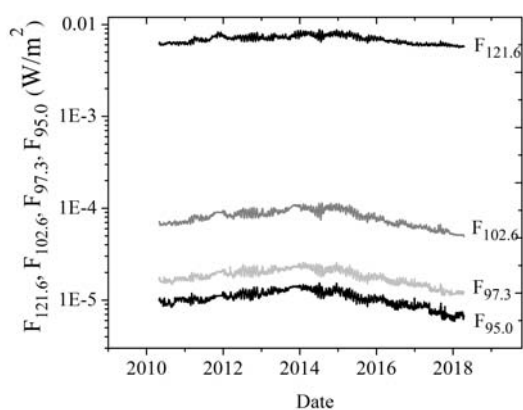
Рис. 1. Вариации излучения Солнца в линиях водорода серии Лаймана в 24 цикле. По оси X – время (годы), по оси Y – поток в Вт/м 2 в логарифмической шкале. Поток в линии L_\alpha на 2–3 порядка больше потоков в других линиях водорода серии Лаймана.
