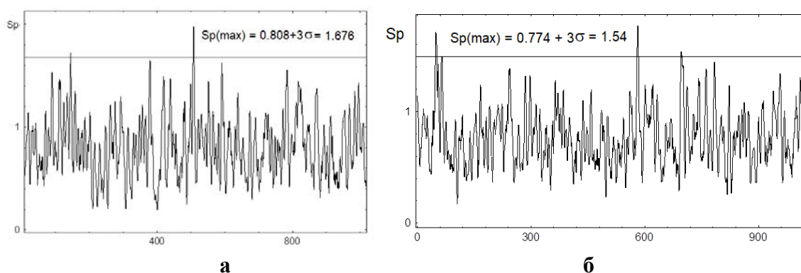
Рис. 1. Спектры мощности 2 мая (а) и 7 мая (б). По горизонтальной оси указаны номера гармоник.
