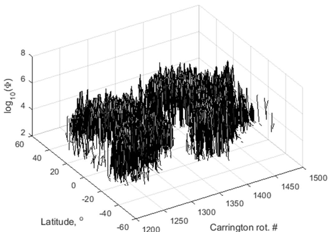
Рис. 1. Диаграмма бабочек в циклах 18 и 19 в масштабе логарифма магнитного потока.
