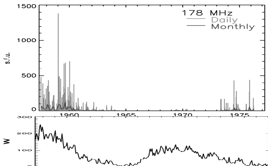
Рис. 1. Временной ряд радиоизлучения Солнца на волне 168 см (вверху) и данные чисел Вольфа за этот период (внизу).
